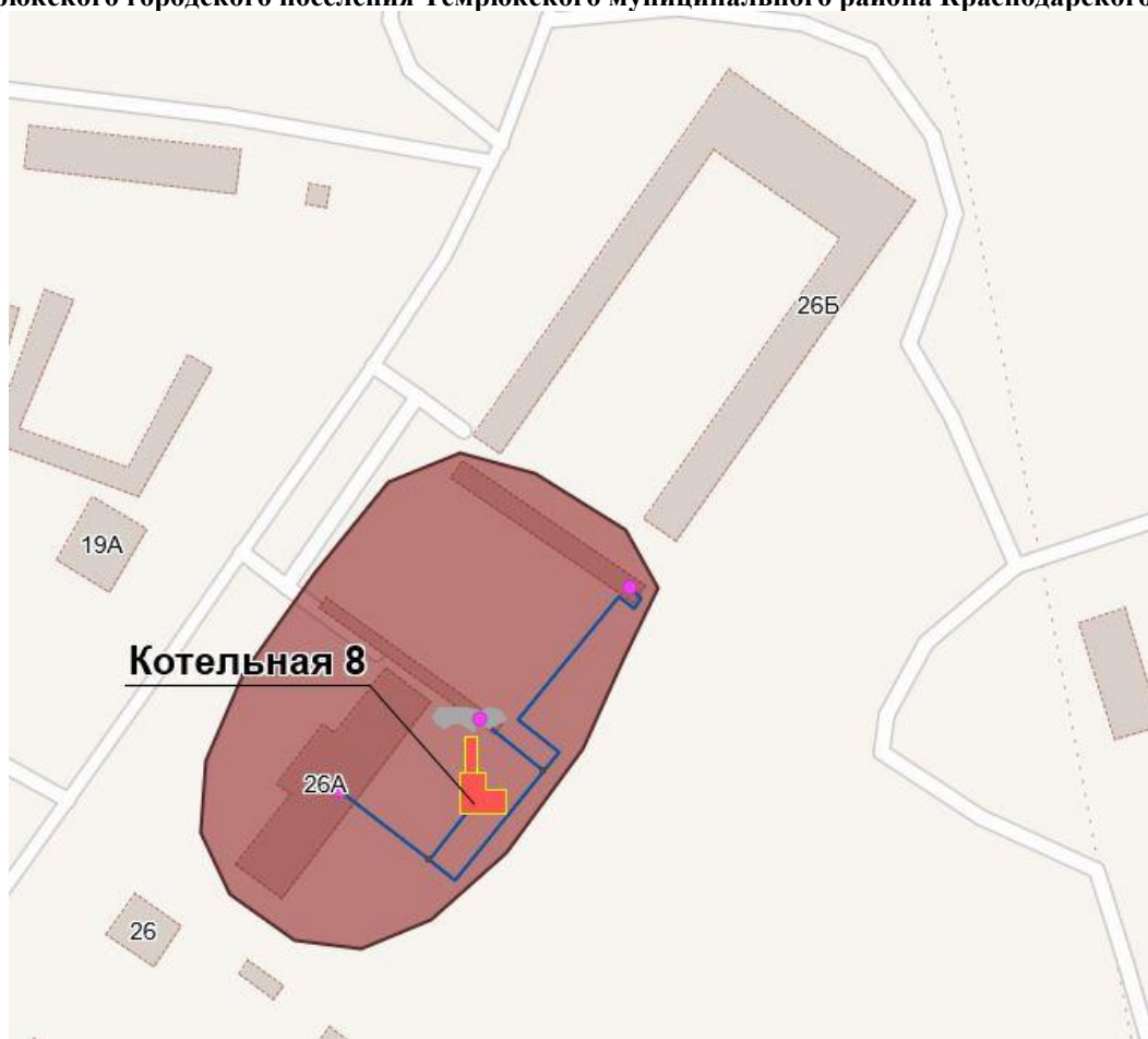
Рисунок 10 Зона действия источника централизованного теплоснабжения (Котельная №8 г. Темрюк, Чужанова, 26к (ТКУ-300) Темрюкского городского поселения Темрюкского муниципального района Краснодарского края
